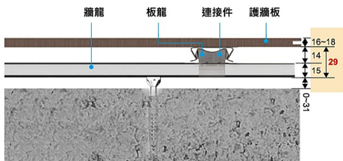
29 牆板系統 俯視圖 零組件請查看 29 牆板目錄
