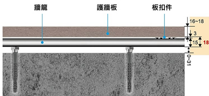
18 牆板系統 俯視圖 零組件請查看 18 牆板目錄
