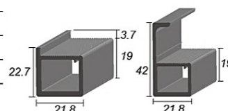
邊框
