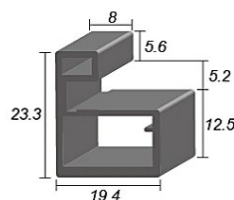
鋁框
