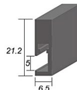
上下框(附左右蓋)
