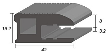
上下鋁橫框
