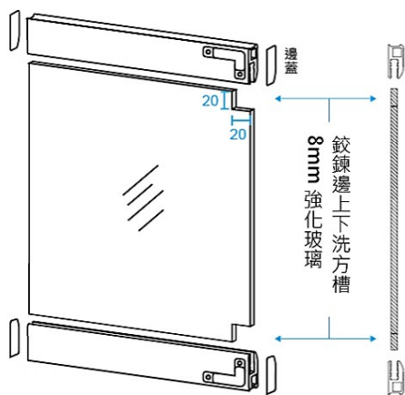
P1 鋁框門背面 組裝圖
