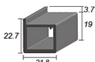
邊框
