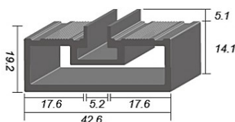
中橫鋁框(搭配活動把手)
