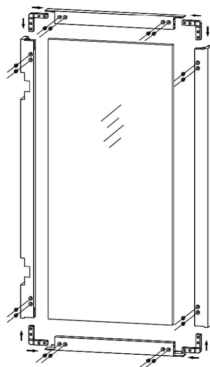
門板背面組裝圖
