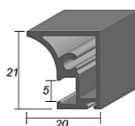
把手框
