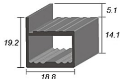
鋁邊框
