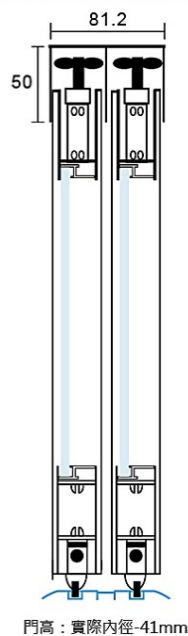
門高：實際內徑-41mm
