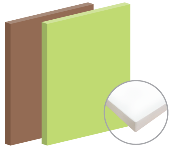
四角無線封邊門板 同心陶烤門板【消光面】 基 材：木芯板 封邊條：同色無線封邊 背 板：純色同心板 同心高光門板【高光面】 基 材：木芯板 封邊條：結晶鋼烤 - 同色無線封邊 背 板：白G美耐板
