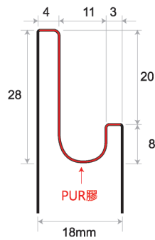
J型門板 木紋門板【浮雕面】x9色 基 材：木芯板 封邊條：同色封邊 背 板：白G美耐板
