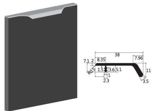
京都型/WP-074(鋁色 / 鈦金色)
