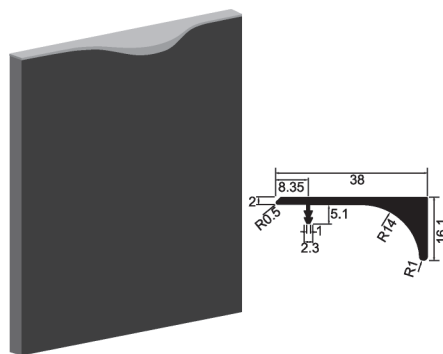
和風型/WP-073(鋁色 / 鈦金色)
