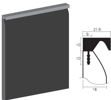
小騎士型/WP-072T(鈦金色)
